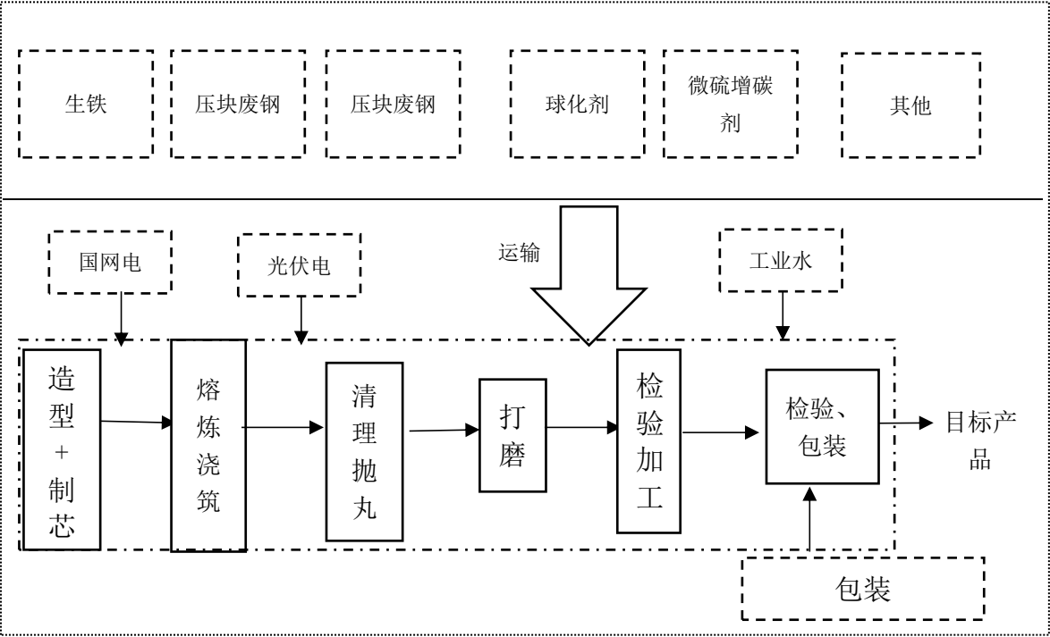
图 1-1 棉纱（40 支）生产系统边界图
